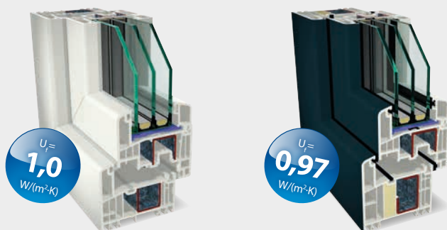
Uski okvir s krilom
