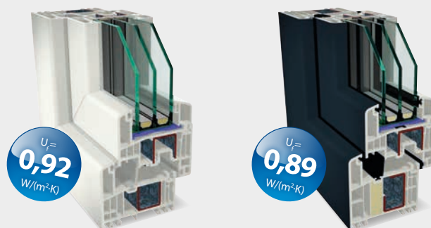
Uski okvir s krilom i ispitanom ift-pogodnosti za pasivne kuće
